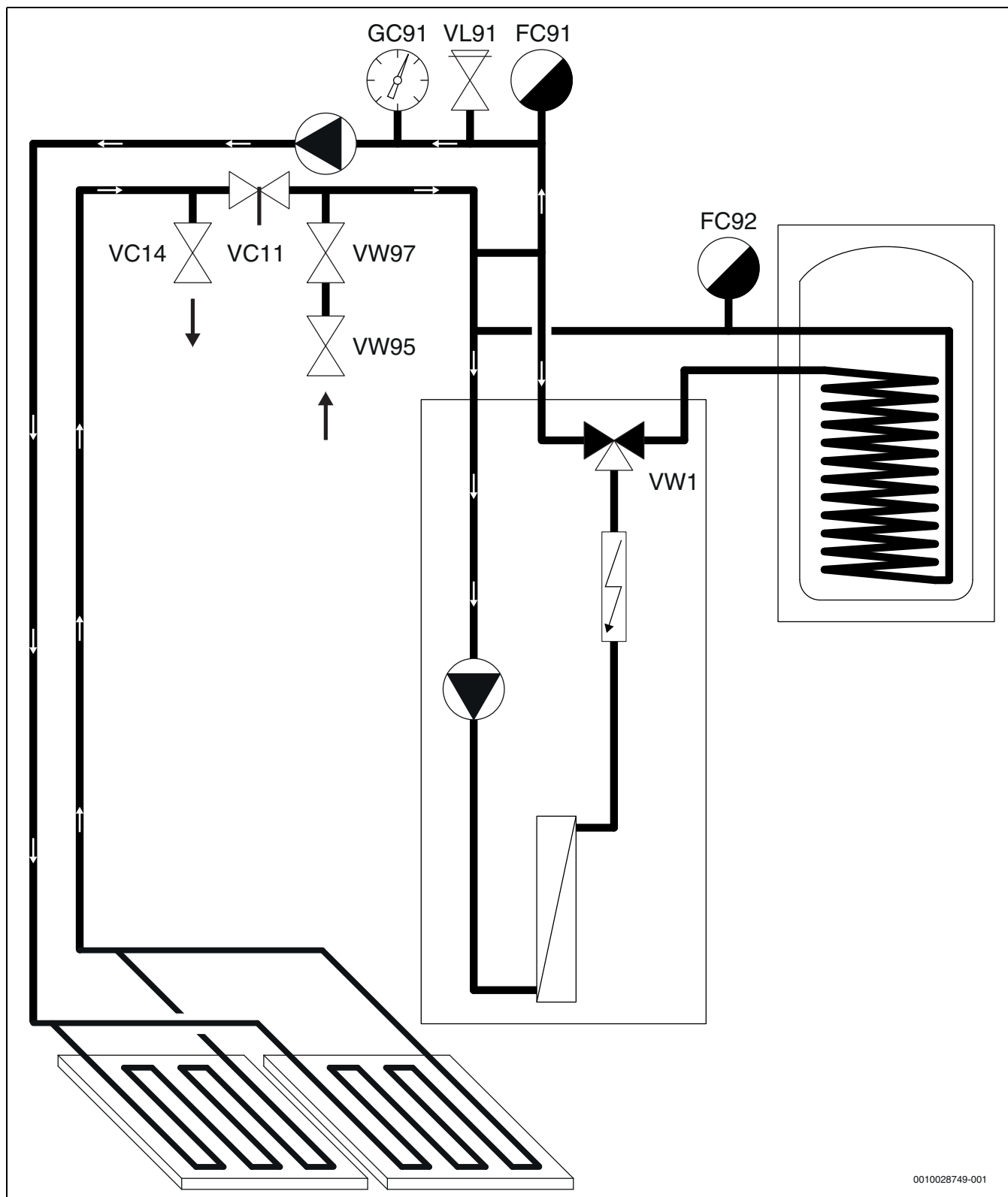
Bild 3 Värmepump och värmesystem med bypass
