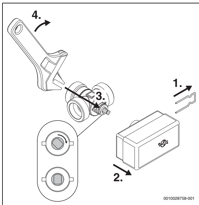
Bild 2 Ventil VW1 i mellanläge
