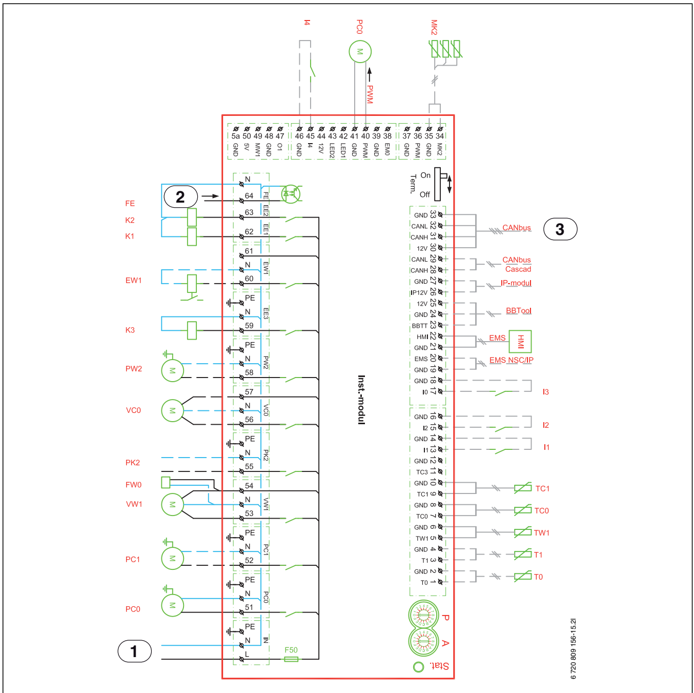
Bild 28 Elschema, Installermodul
