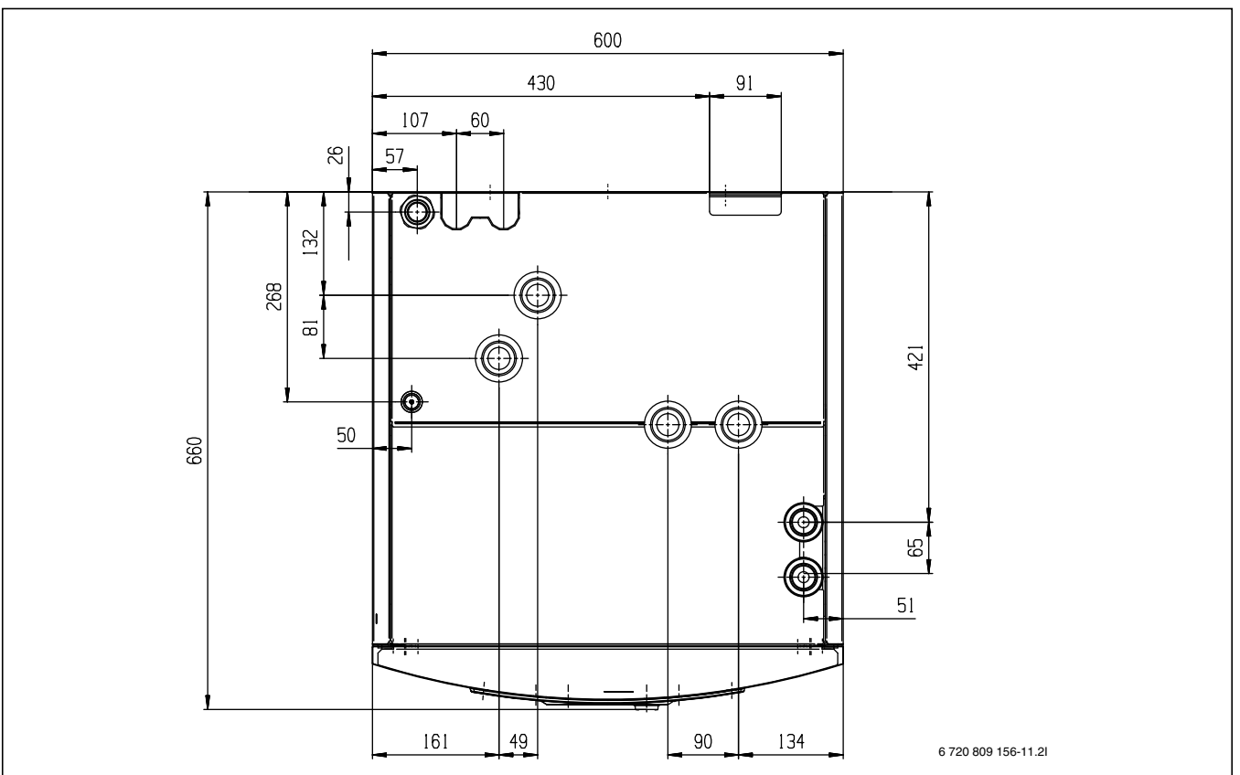
Bild 7 Mått takvy
