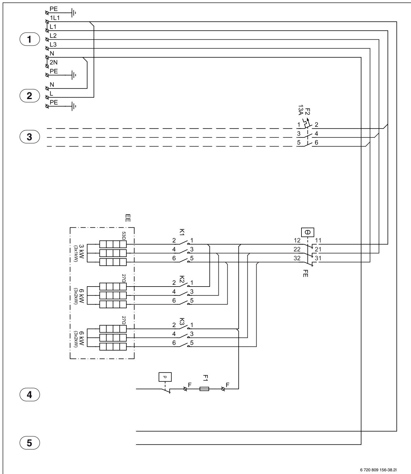
Bild 27 Elmatning värmepump och värmepumpsmodul 15kW
