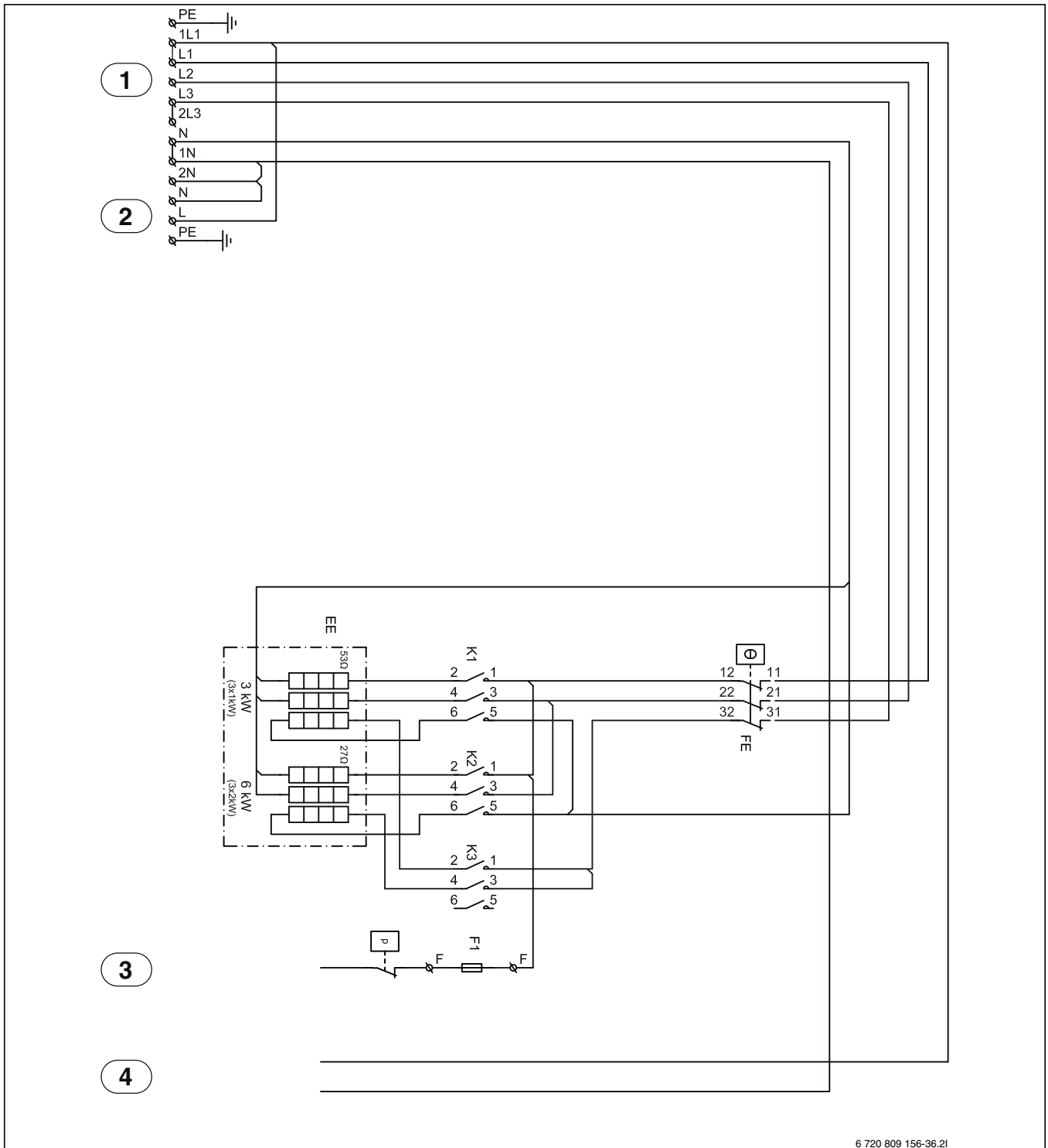
Bild 26 Elmatning värmepump och värmepumpsmodul 9kW
