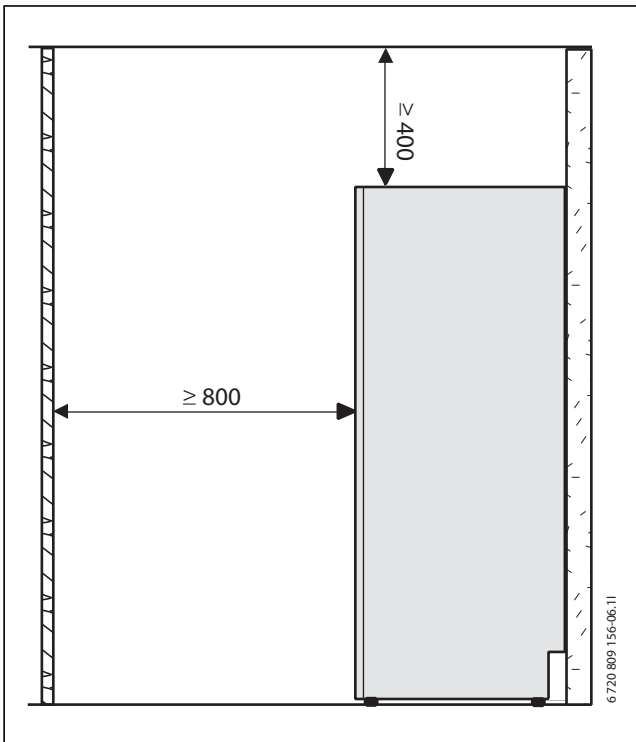
Bild 5 Minimiavstånd värmepumpsmodul
