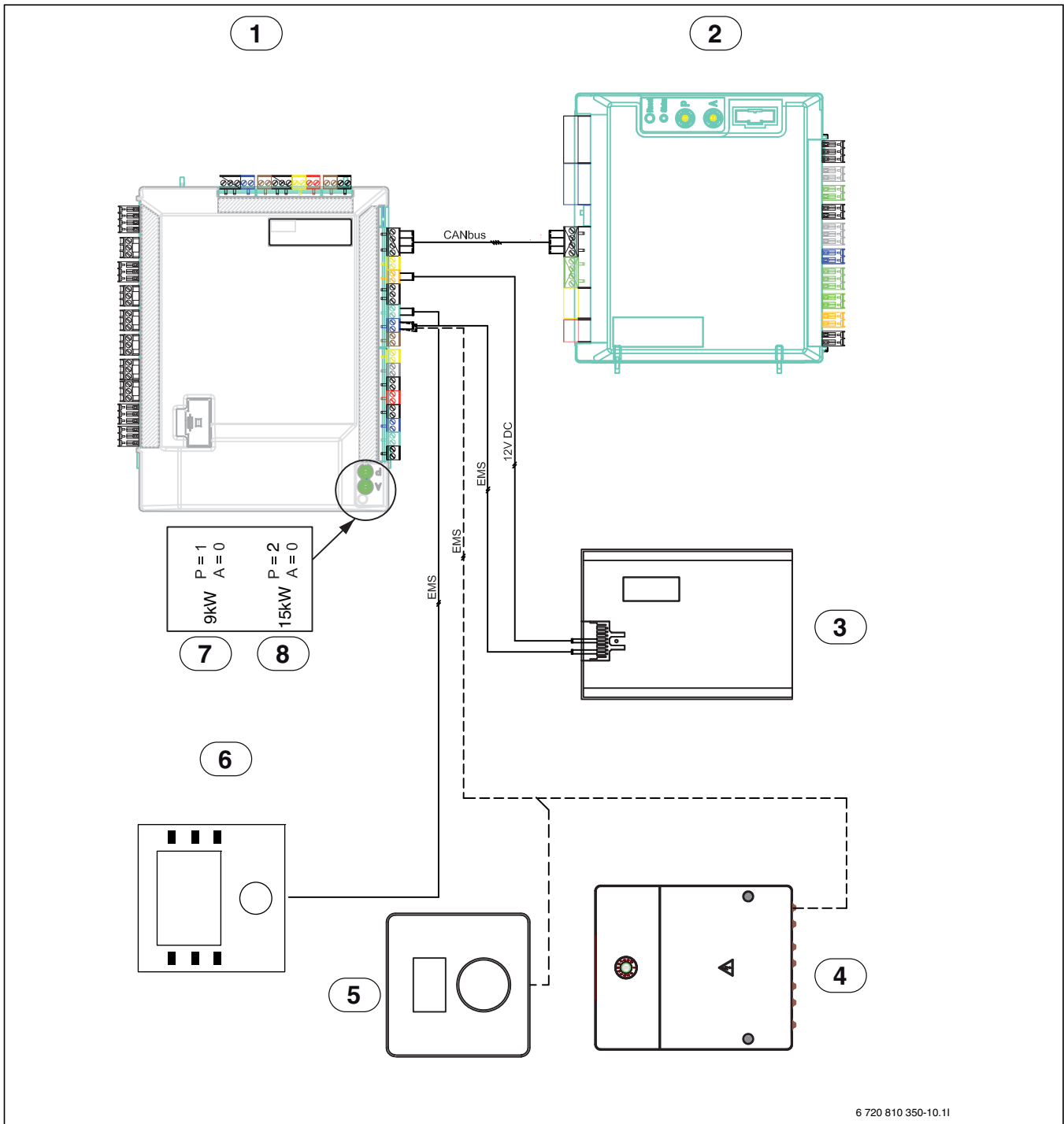
Bild 29 Kretsschema värmepump/värmepumpsmodul
