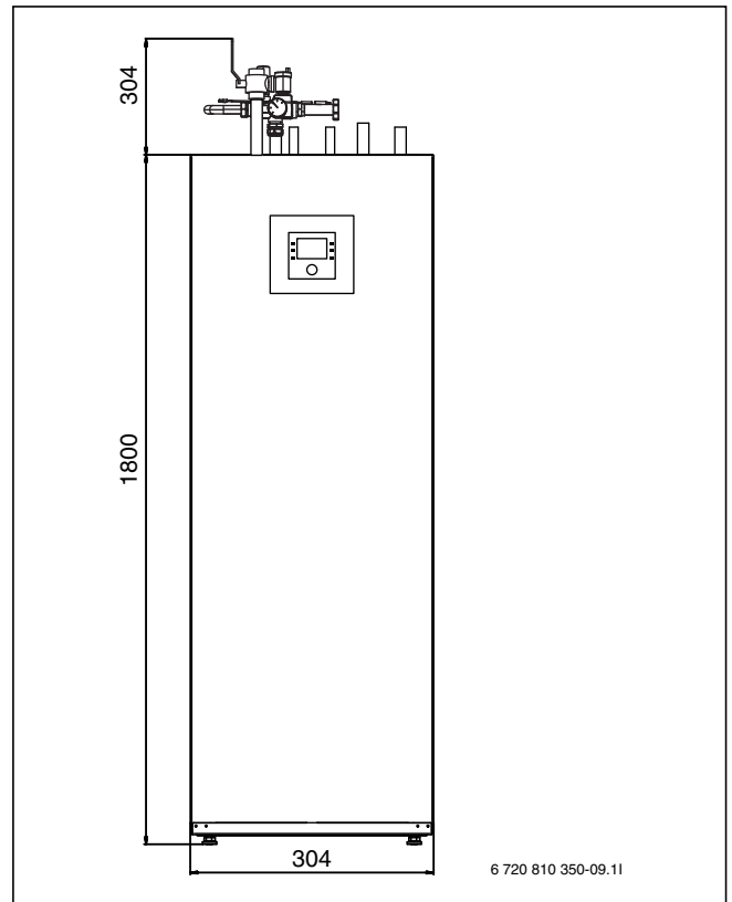
Bild 6 Mått värmepumpsmodul (mm)
