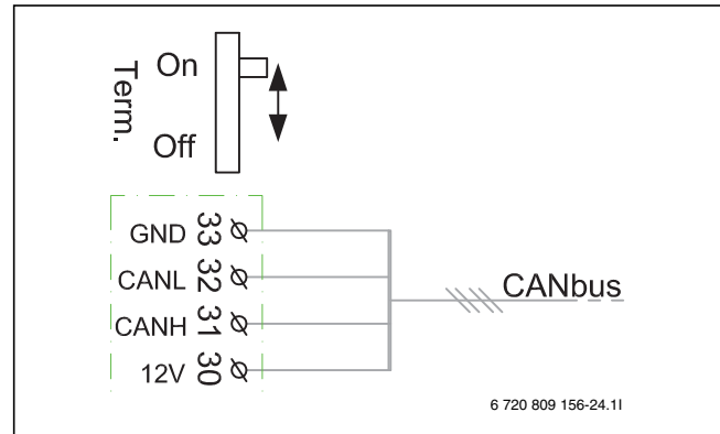
Bild 17 Terminering CAN-BUS
