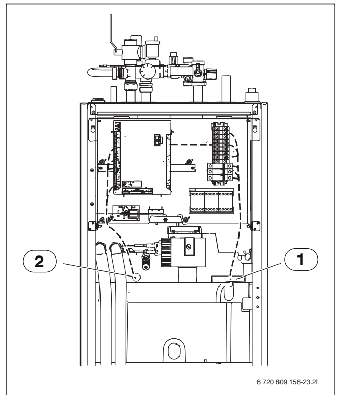
Bild 19 Kabelgenomföringar
