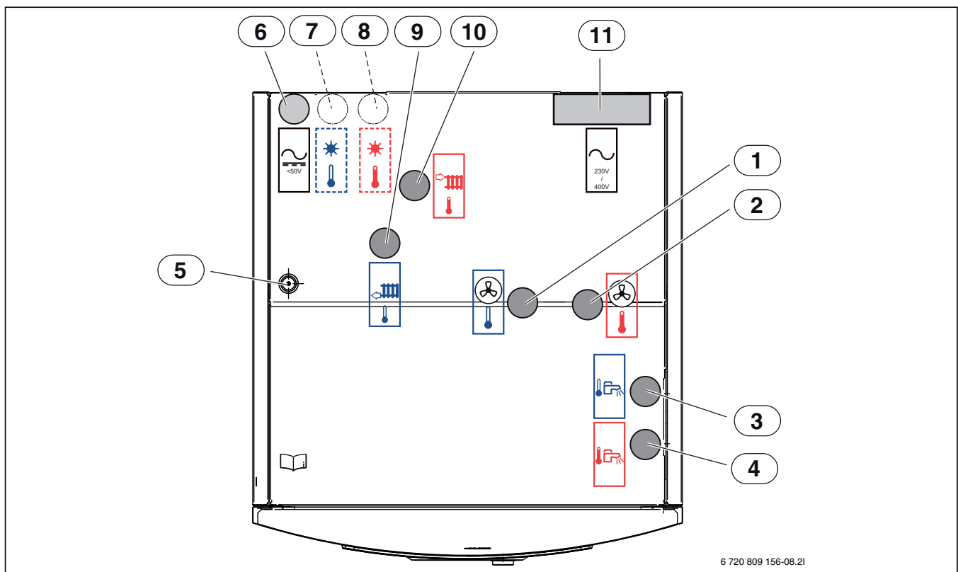
Bild 8 Värmepumpsmodul anslutningar
