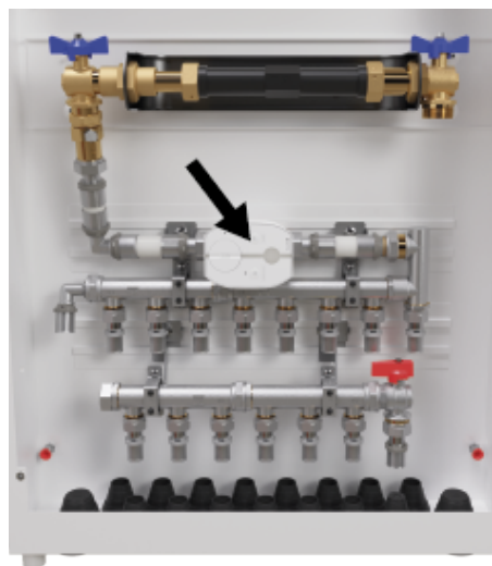
Vattenfelsbrytaren monterad i skåpet.
